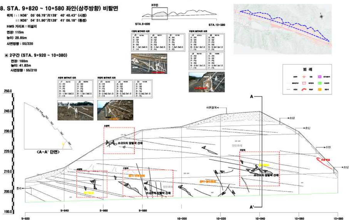
[그림 37.14] 상주절토37 검토대상 비탈면구간
